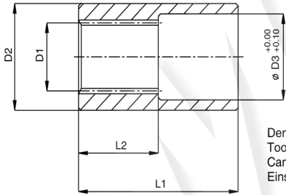
Dentatura su due lati Toothting on two sides Cannelure sur deux côté Beidseitig verzahnt
